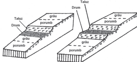
Fig. 3. Drumuri agricole sau tehnologice
