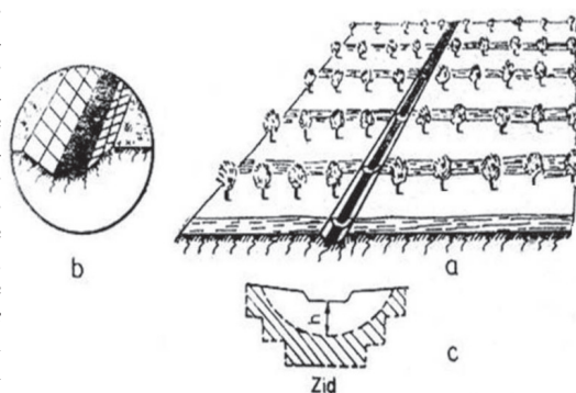
Fig. 4. Debușeu într-o livadă terasată cu căderi consolidate: a - vedere generală; b - debușeu datat; c - cădere consolidată
