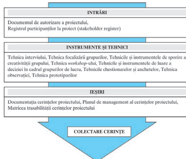
Fig.2. Intrări, instrumente, tehnici și ieșiri specifice procesului de colectare a cerințelor
